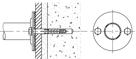
DETALLE A E= 1:3
